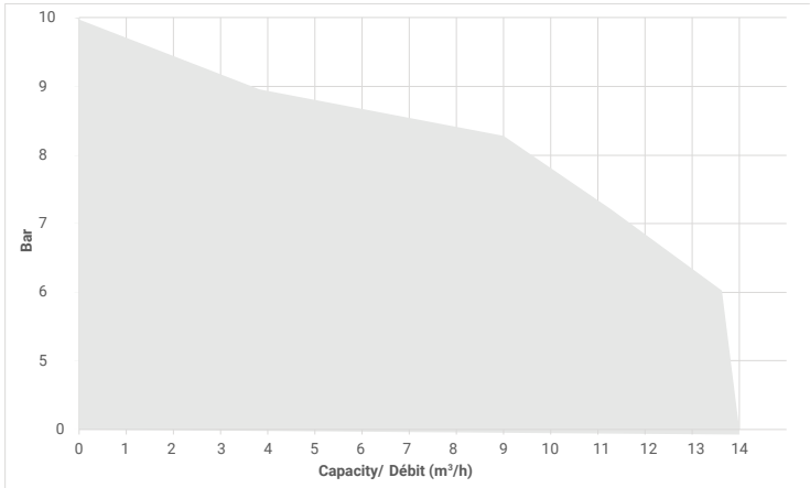
Characteristic curve / Courbe caractéristiques
